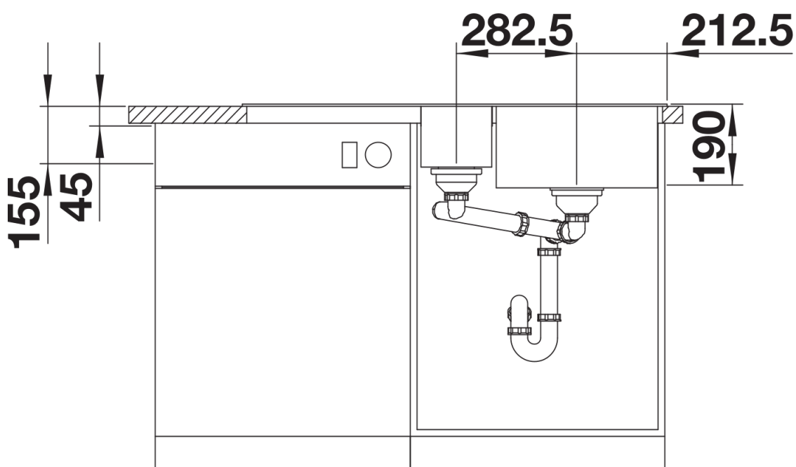
Frontansicht
